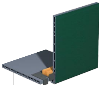
Overstekplafond met dakrandpaneel en montageclip 10 mm 2845
