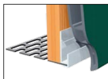
Inhaak startprofiel 2808
